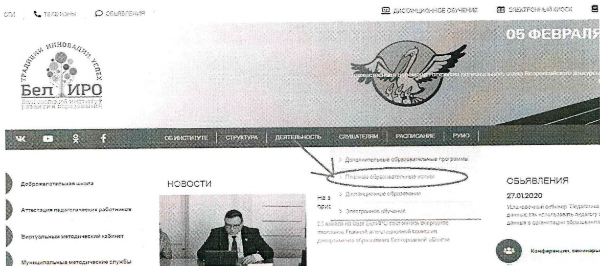
Рис. 1. Раздел «Слушателям»
