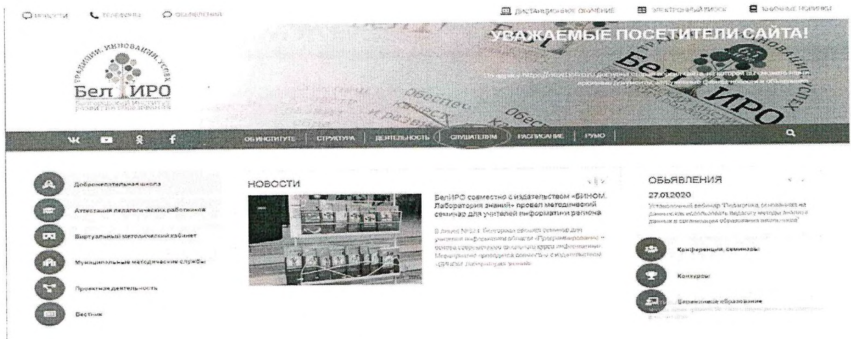
Рис. 1. Раздел «Слушателям»
